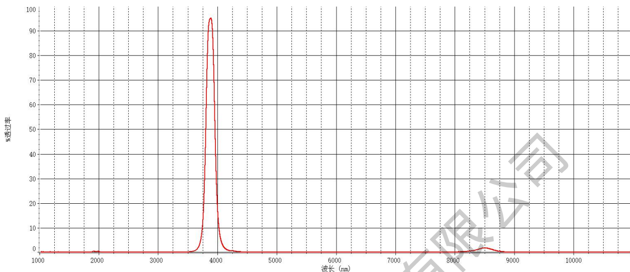
3. 85um 红外窄带滤光片透射曲线图
